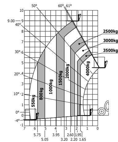
Laaddiagram ruw terrein (EN 1459 B)
