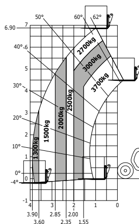
Laaddiagram ruw terrein (EN 1459 B)
