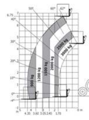
Laaddiagram ruw terrein (EN 1459 B)
