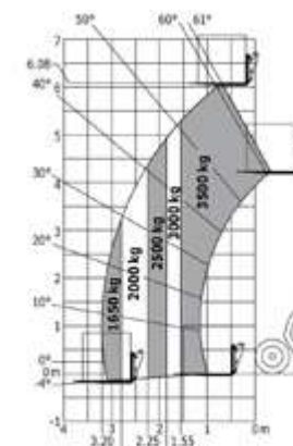
Laaddiagram ruw terrein (EN 1459 B)
