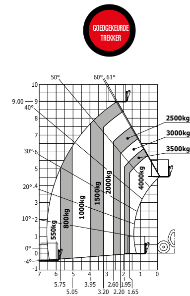
Laaddiagram ruw terrein (EN 1459 B)
