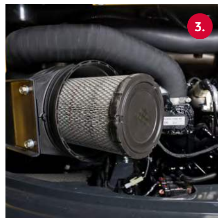
3. Luchtfilter 6. Brandstofpomp
