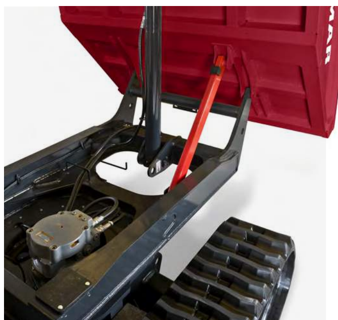
WAGEN MET KLEPPEN AAN DRIE ZIJDEN, STORTEN AAN ACHTERZIJDE
